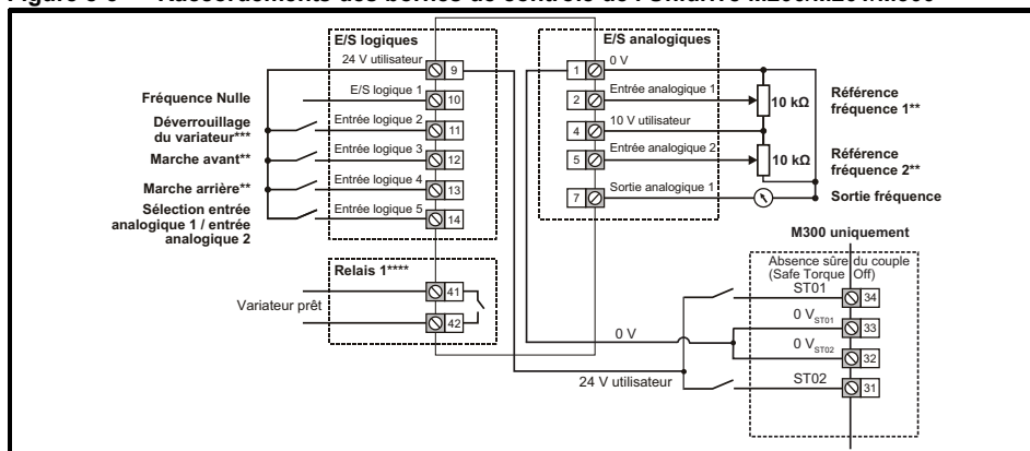
Figure 8-3 Raccordements des bornes de contrôle de l'Unidrive M200/M201/M300
