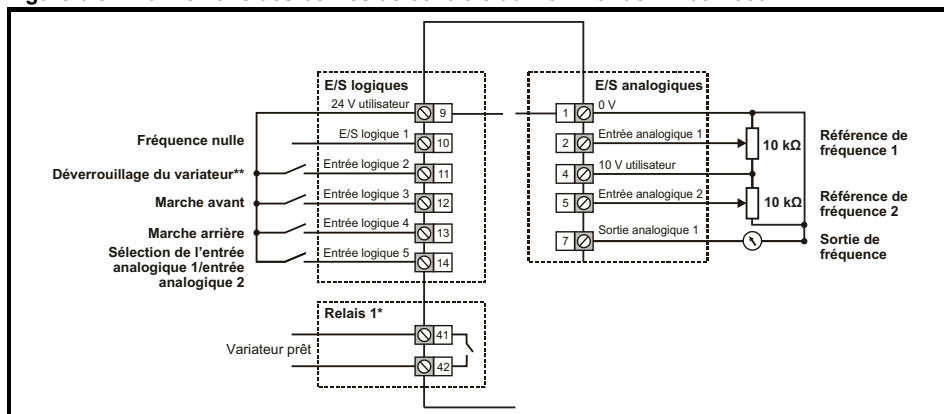
Figure 6-3 Connexions des bornes de contrôle du Commander C200/C300
