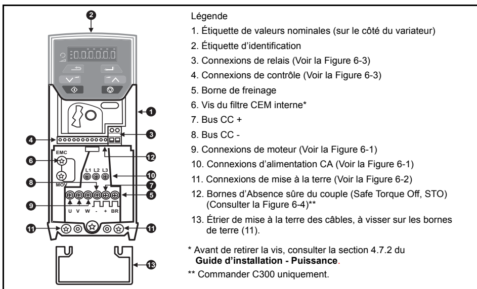
Figure 1-1 Schéma des fonctions (taille 2 illustrée)
